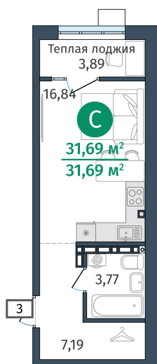
План квартиры
